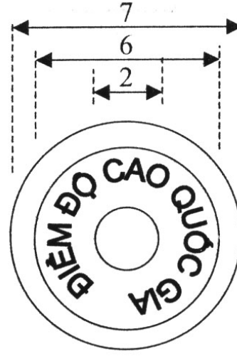
Hình 8: Dấu kim loại
