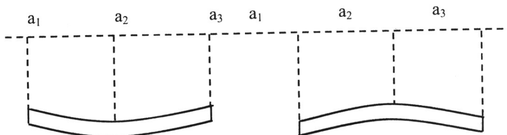
Hình vẽ đặt mia inva nằm nghiêng để kiểm tra độ vồng
