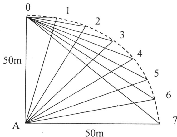
Hình vẽ bãi kiểm nghiệm theo yêu cầu 2
