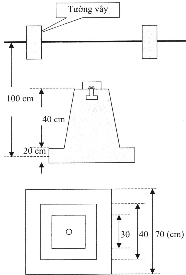
Hình 4: Móc thường trên vỉa đá ngầm
