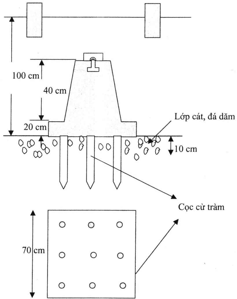
Hình 6: Mốc chân tường
