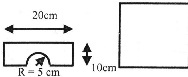
Hình 10: Mặt móc độ cao
