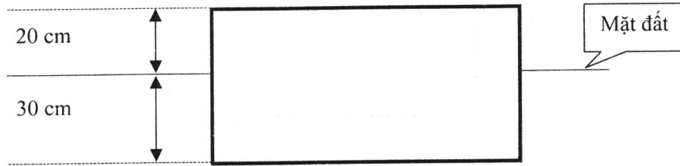
Hình 11. Quy cách tường vây mốc cơ bản
