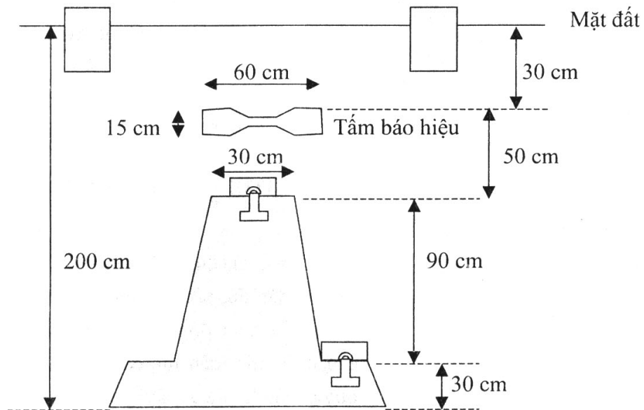
Hình 1: Móc cơ bản chôn chìm
