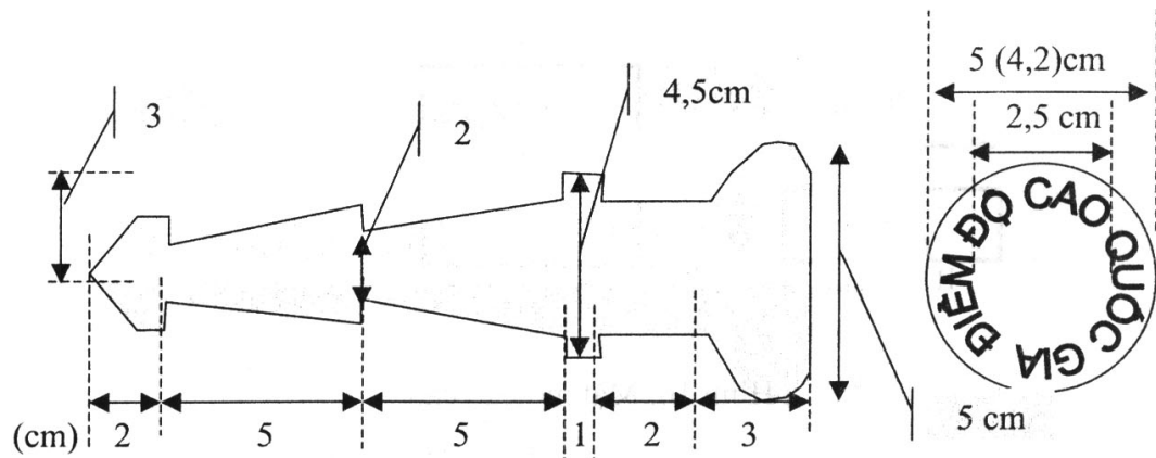
Hình 6: Mốc chân tường
