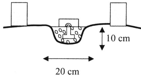
Hình 5: Móc thường vùng đất yếu
