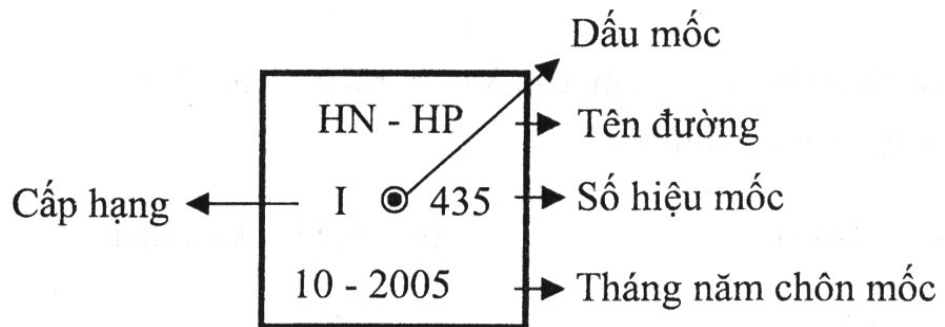
Hình 10: Mặt móc độ cao
